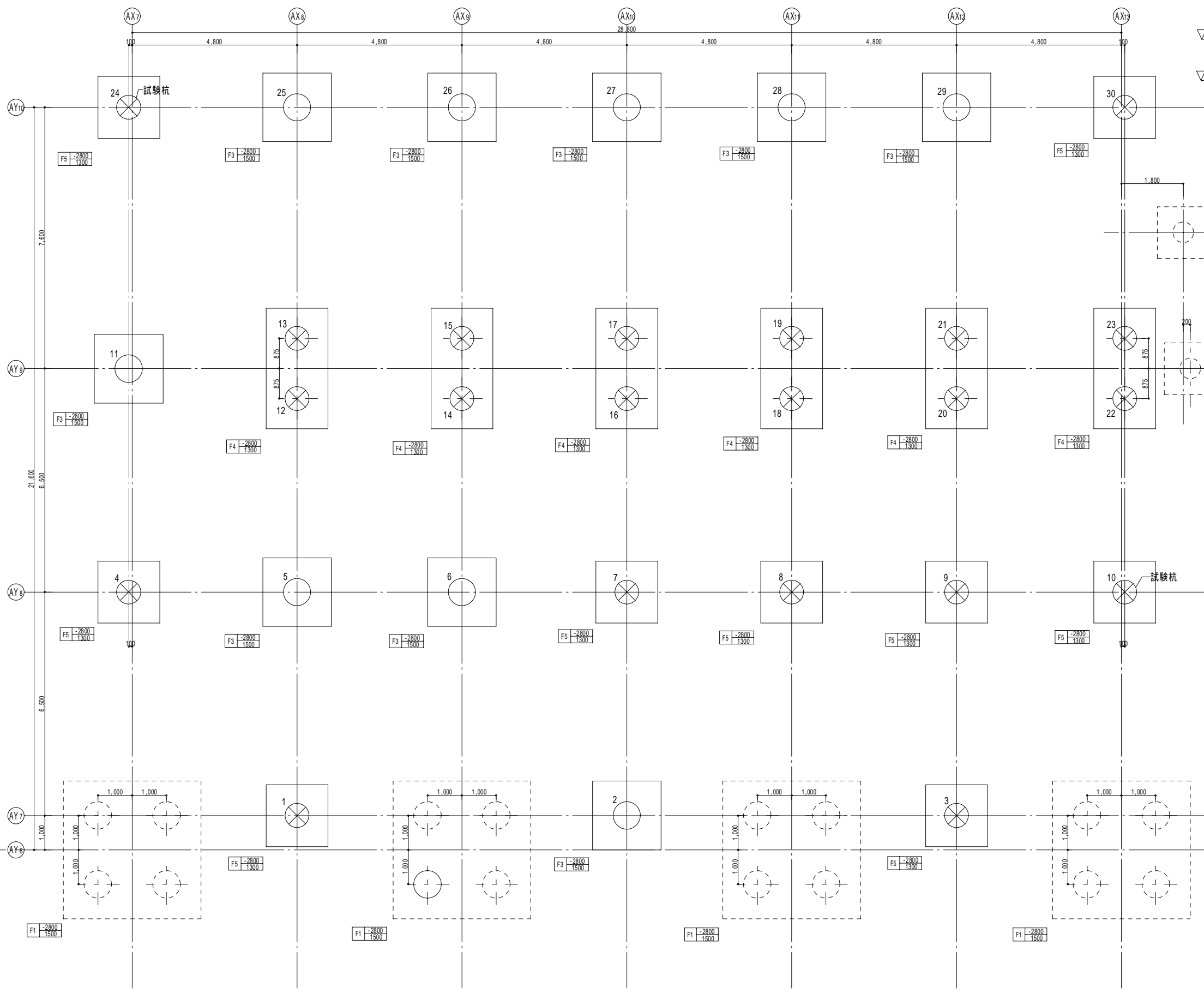
杭伏せ図
